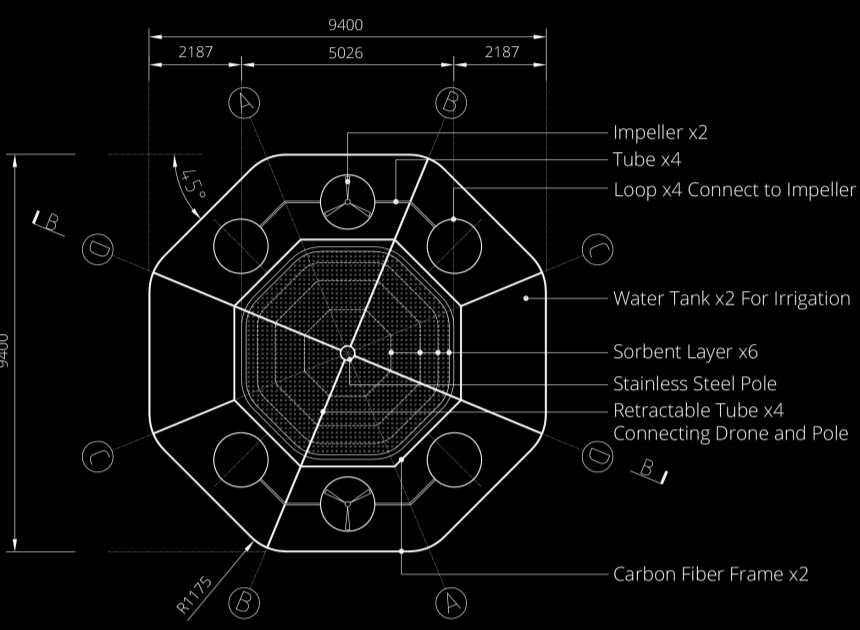
A-A Section
