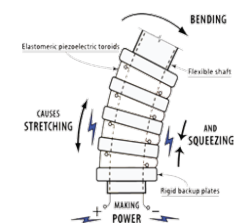
2 PIEZOELECTRIC POLES
